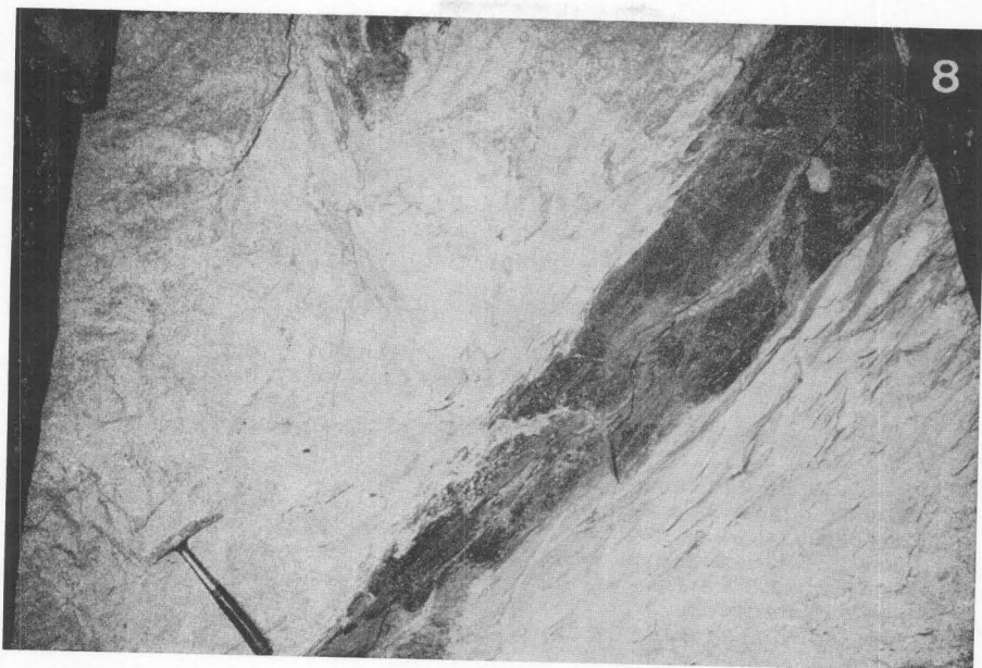
8. Fascia di scisto ad albite, talco, clorite, muscovite, con accessori vari, nel talco
