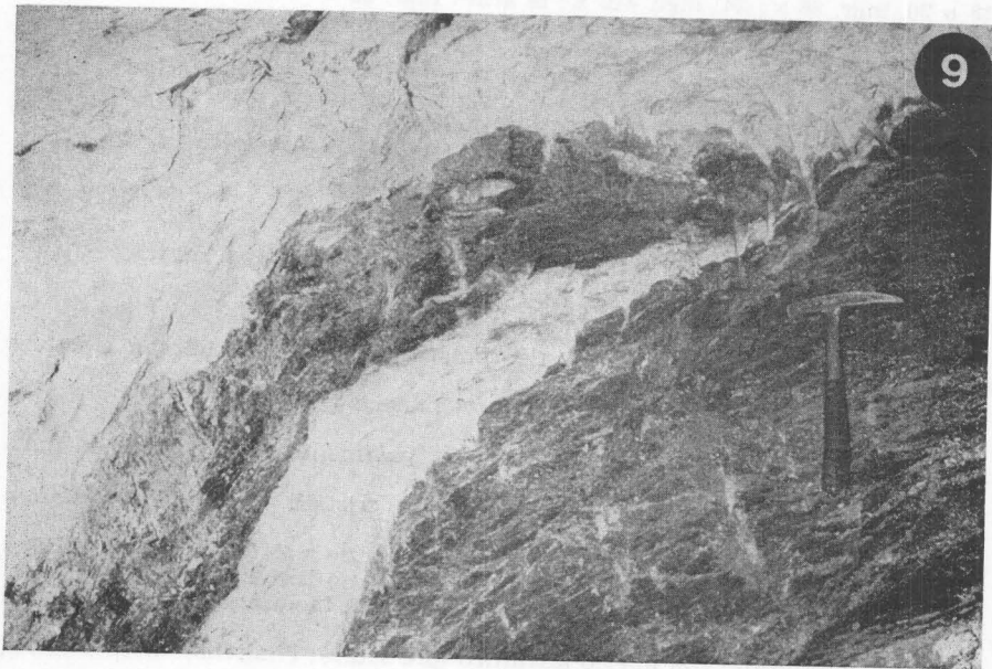
9. Mica-cloritescisto ad epidoti cloritoide, granato (scuro) nel talco
