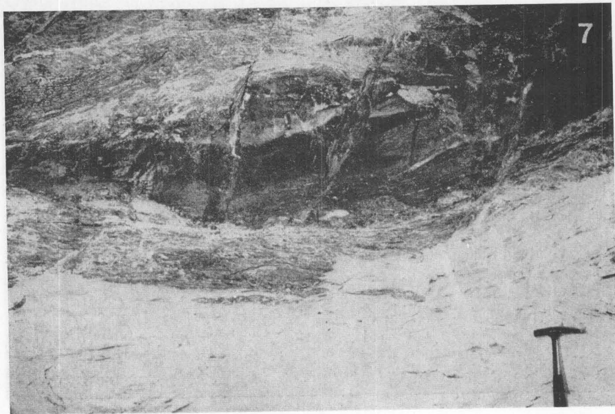
7. Lente di scisto ovoiditico (scuro) nel talco frammisto a clorite e passante a mica-cloritescisto; in basso, talco bianco
